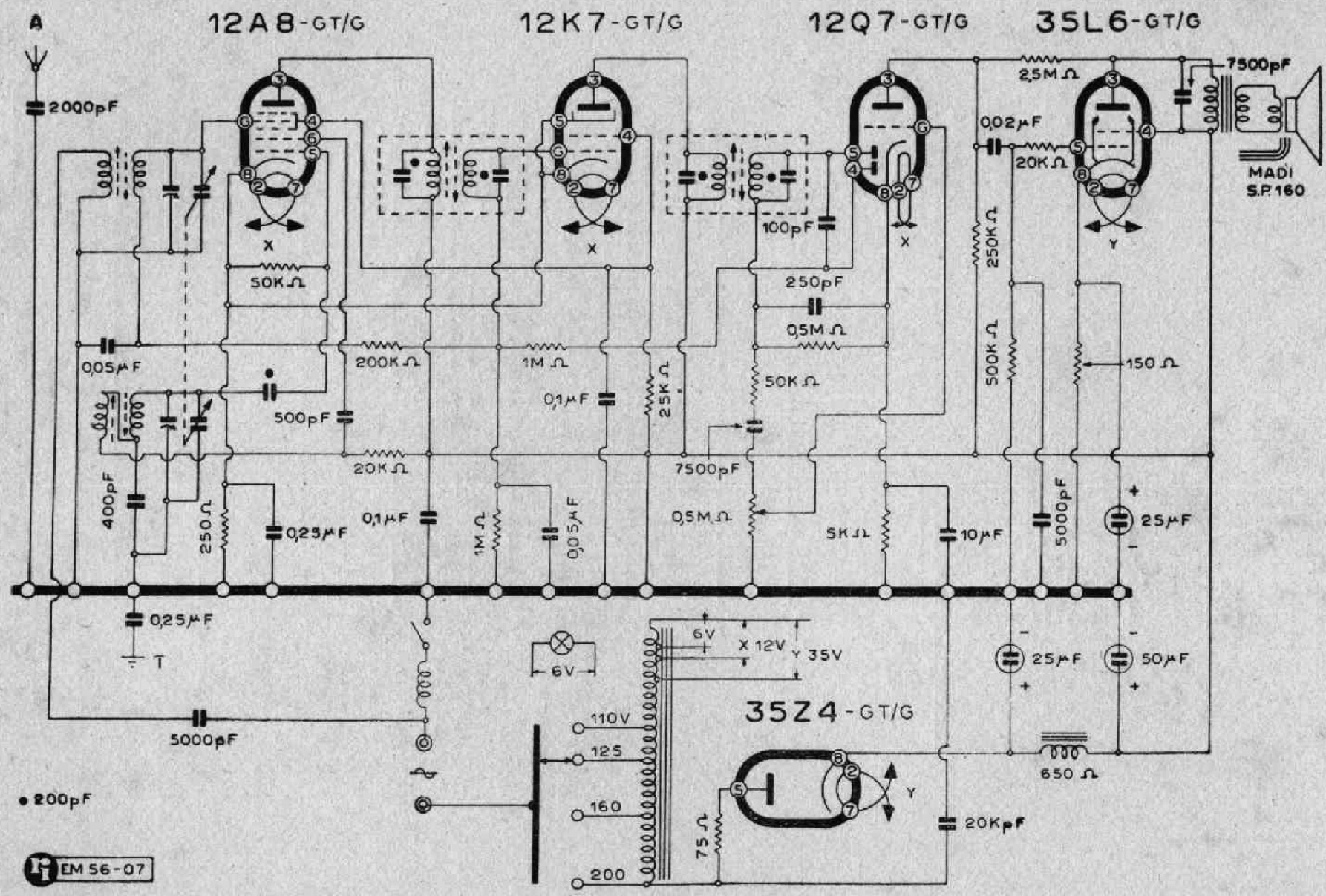
Lo schema elettrico del mod. AR 48
